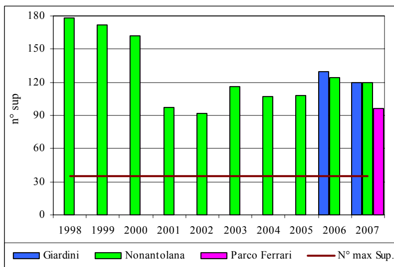
Figura 1.7: PM10 - trend dei superamenti del VL
