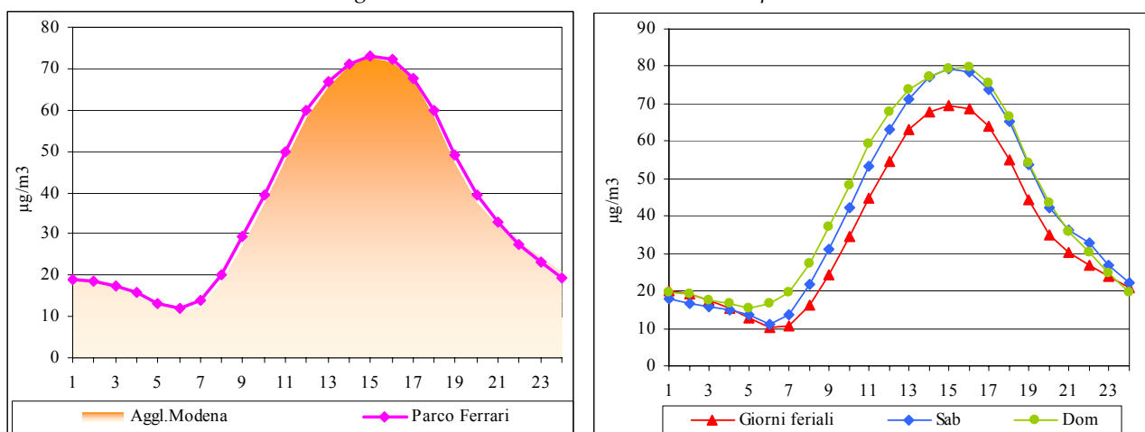
Figura 1.15: O 3 - giorno tipico annuale e giorno tipico feriale e festivo
