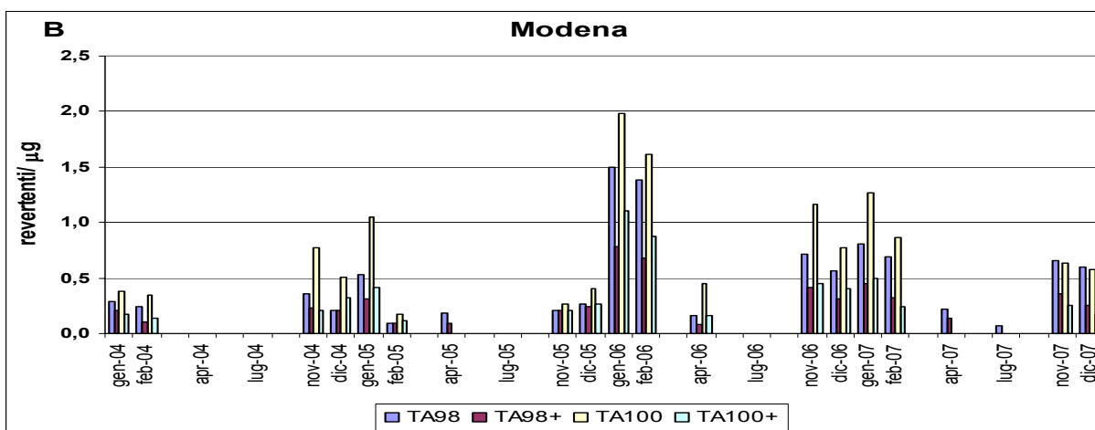
Figura 8.3: Evoluzione temporale della genotossicità del particolato atmosferico urbano (PM 2,5 ) rilevata attraverso l'induzione di revertenti/Nm 3 (A) e revertenti/μg polveri (B) in Salmonella typhimurium ceppi TA98 e TA100 con (+) e senza attivazione metabolica esogena.
