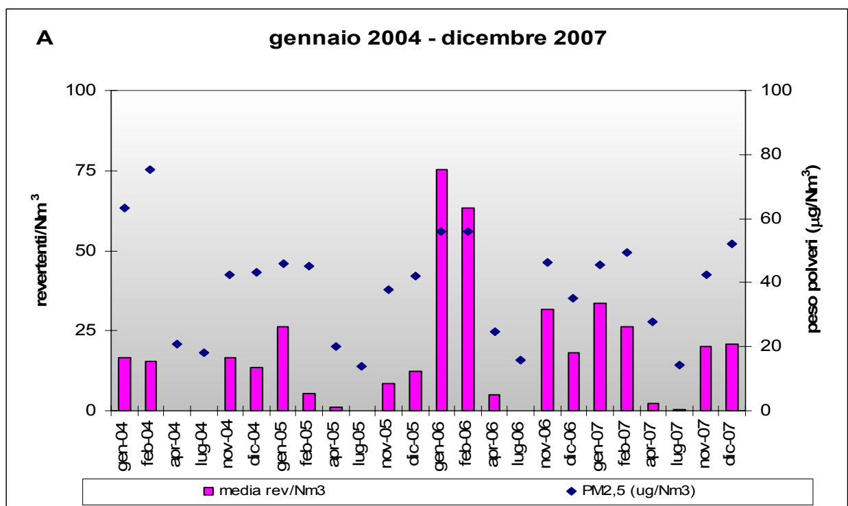
Figura 8.2: Andamenti della mutagenicità del PM 2,5 , espressa come sommatoria dei revertenti/Nm 3 indotti da estratti di campioni mensili, e delle concentrazioni (medie mensili) delle polveri.
