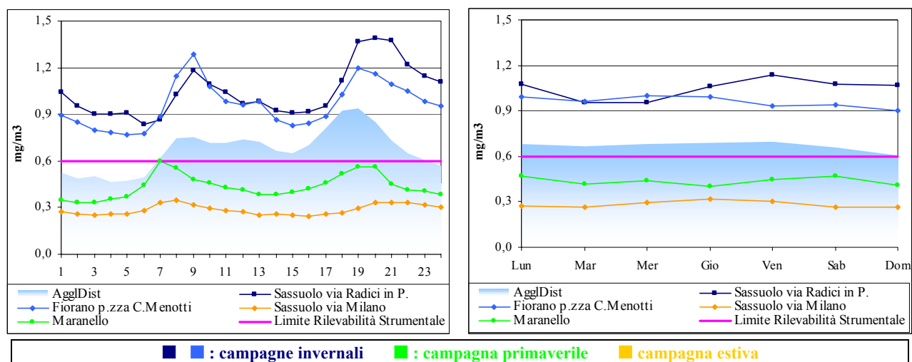
Figura 4.5:CO - giorno tipico settimana tipica nei diversi periodi di monitoraggio
