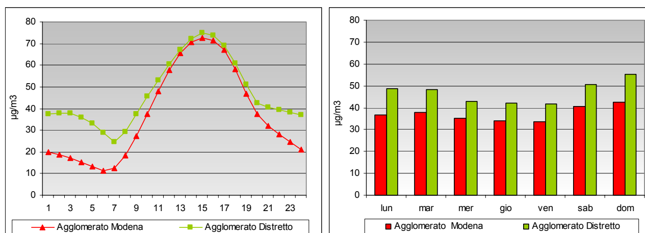
Figura 4.15: O3 - giorno tipico e settimana tipica annuale
