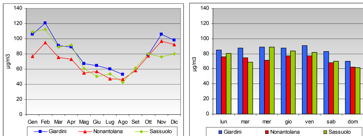
Figura 4.7: PTS - medie mensili e settimana tipica annuale
