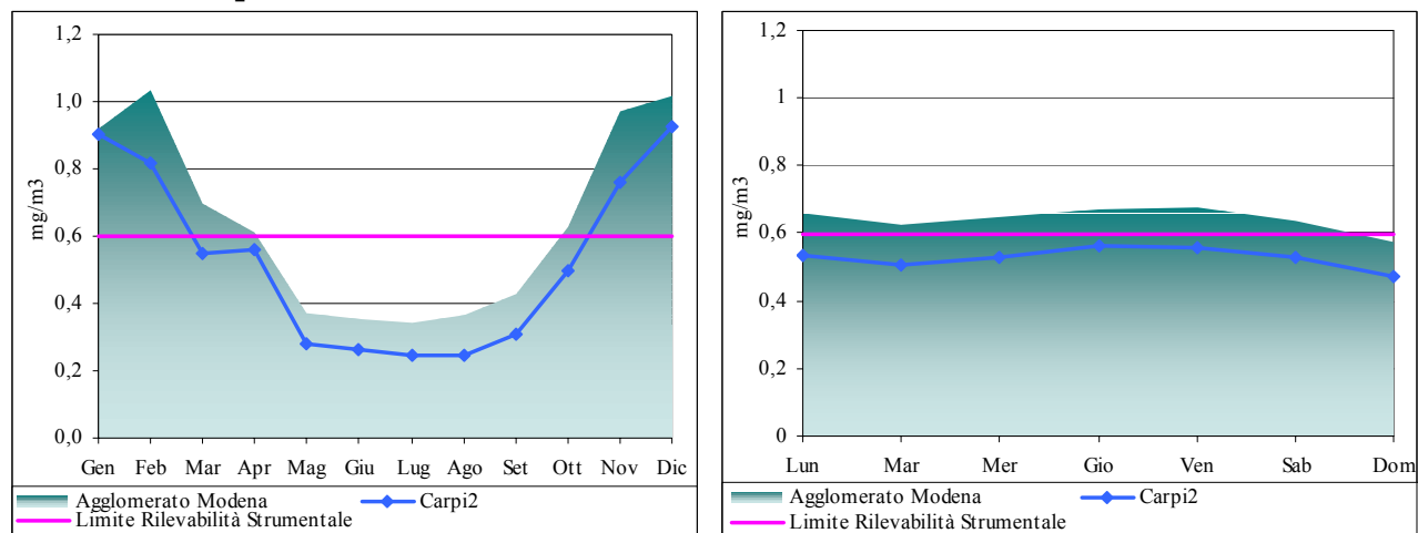
Figura 2.6: CO - concentrazioni medie mensili e settimana tipica annuale
