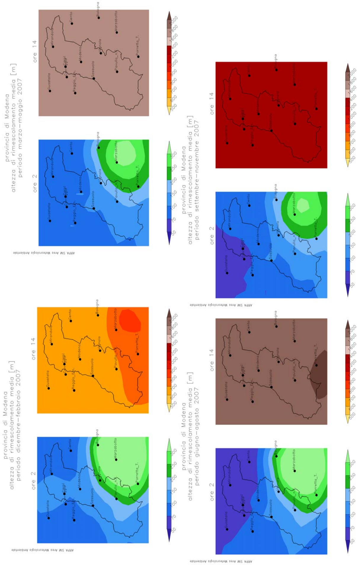
Figura 2.6- Altezza di rimescolamento media nei quattro trimestri dell'anno sul territorio provinciale (dati CALMET)
