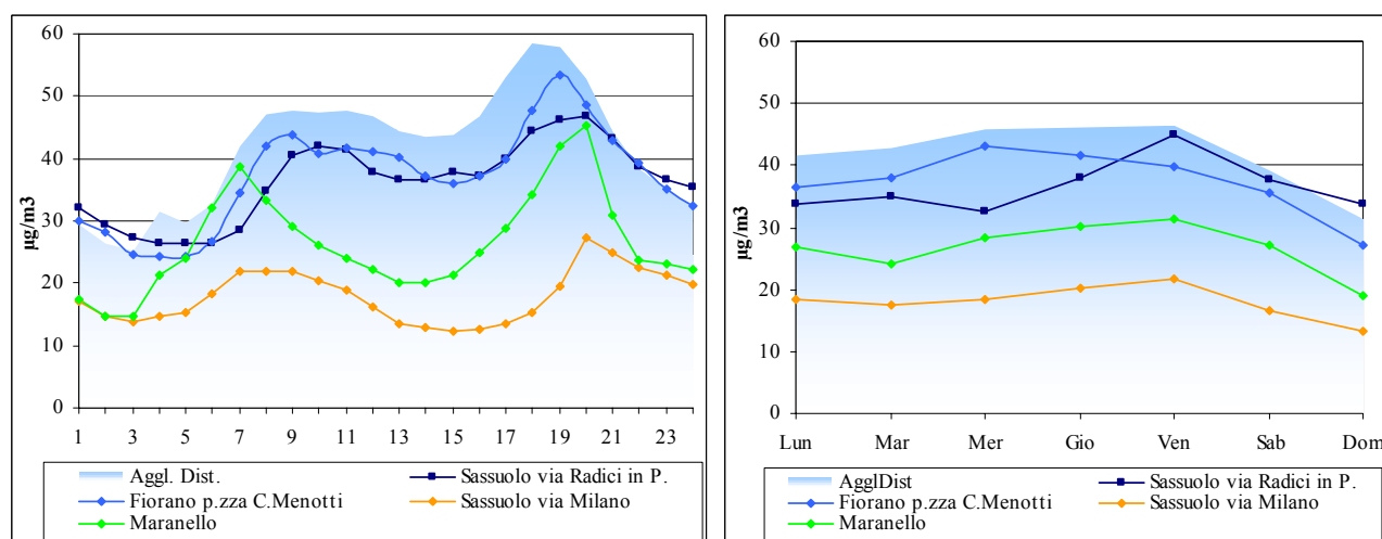
Figura 4.1:NO 2 - giorno tipico e settimana tipica nei diversi periodi di monitoraggio
