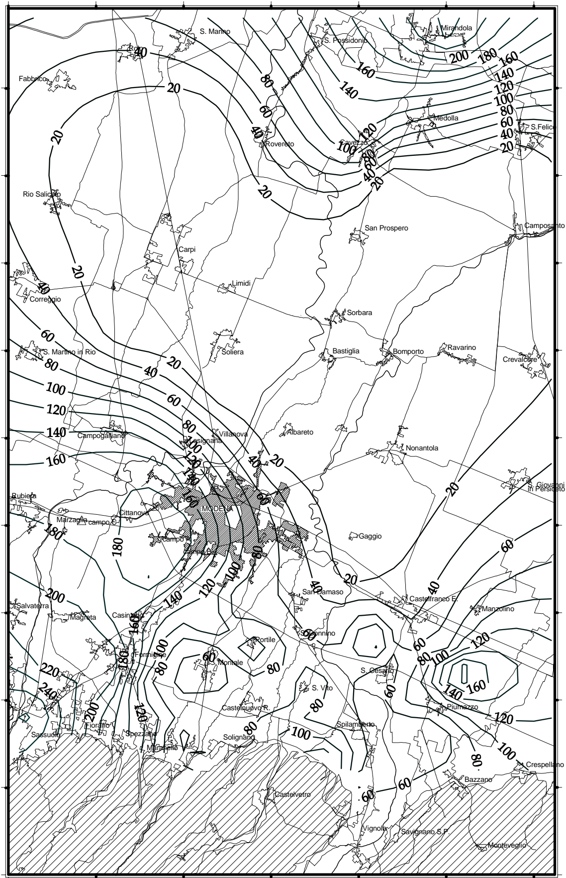
Figura 19 - Solfati (mg/l) media anno 2004.
