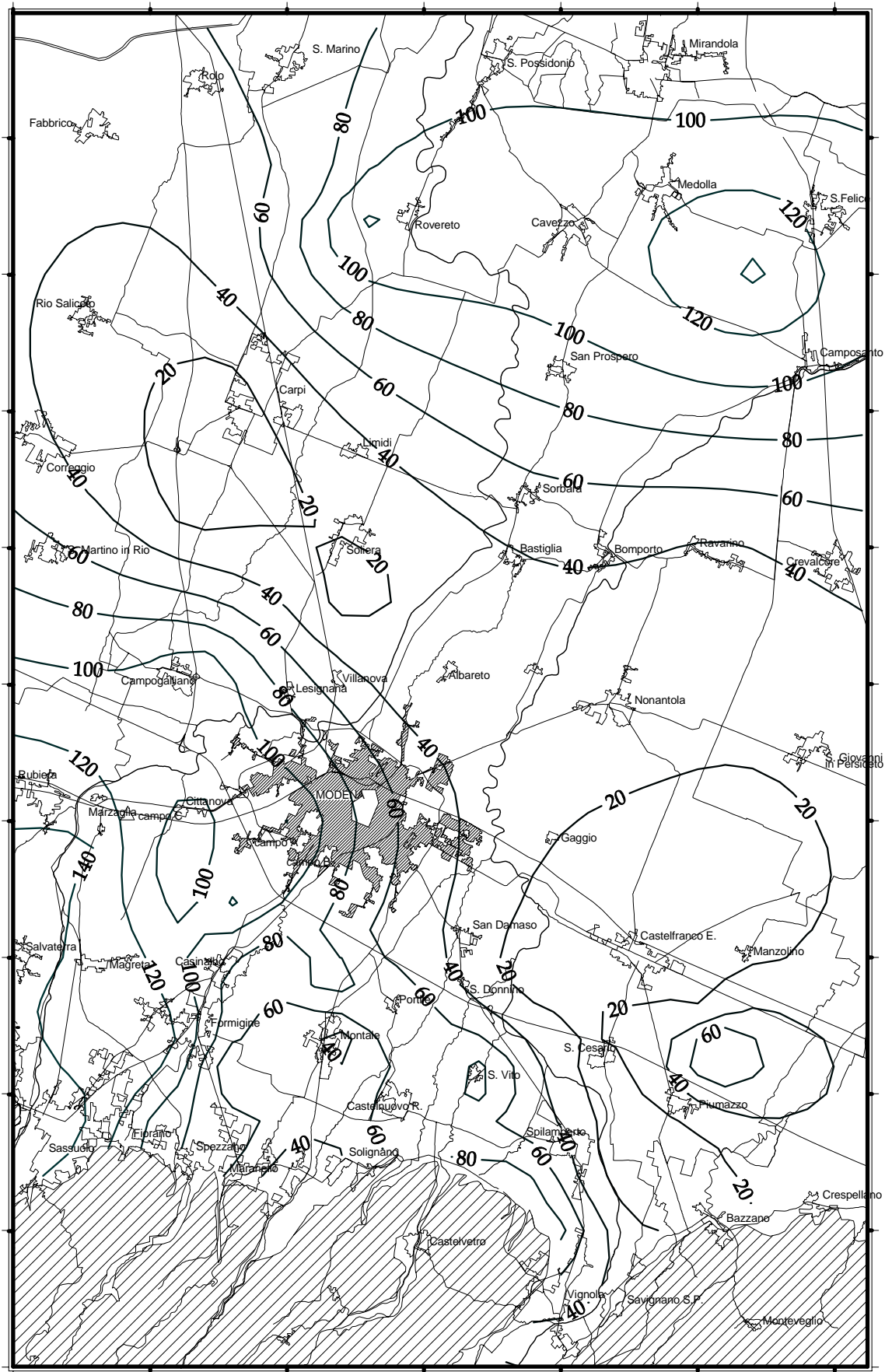
Figura 20 - Cloruri (mg/l) media anno 2004.
