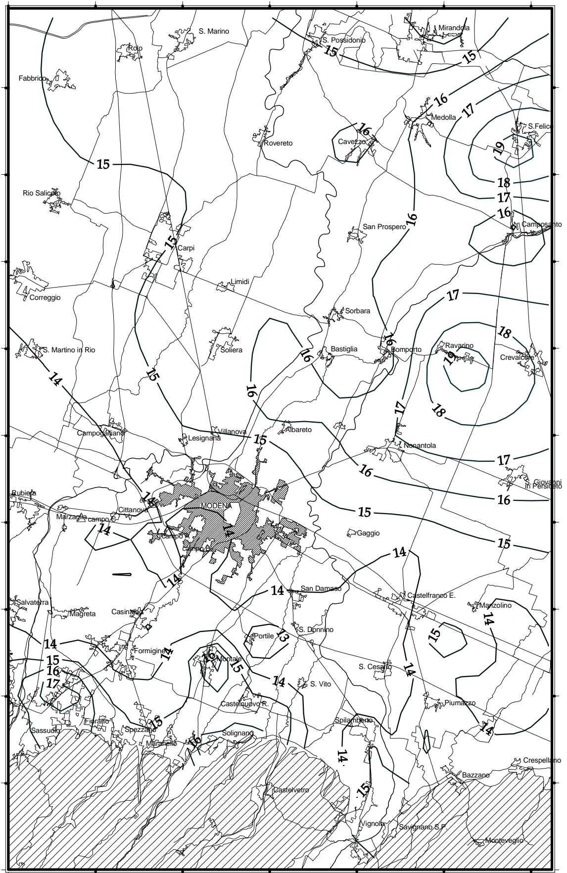
Figura 16 - Temperatura (°C) media anno 2004.
