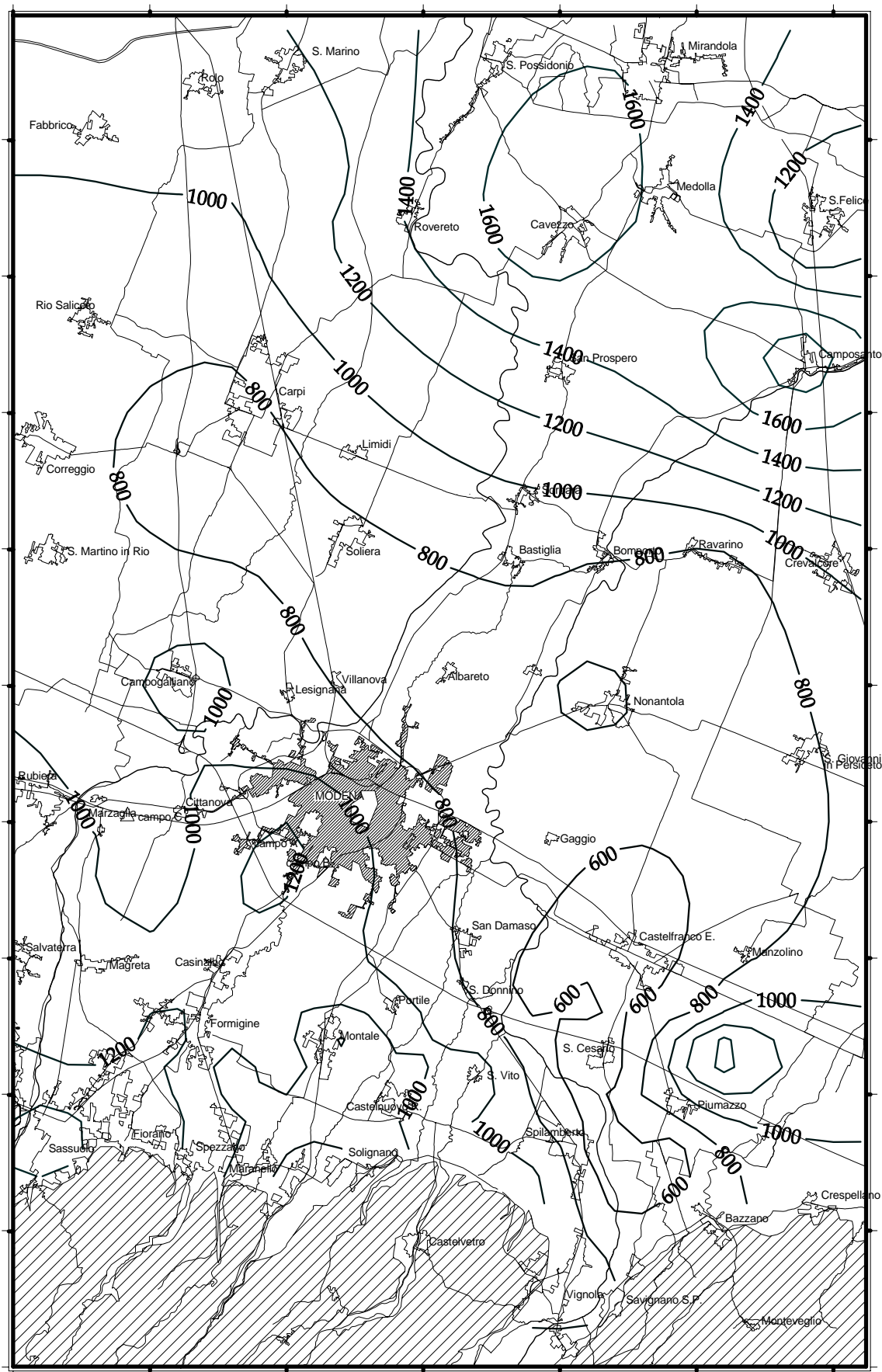
Figura 17 - Conducibilità ( \mu\text{S}/\text{cm} ) media anno 2004.
