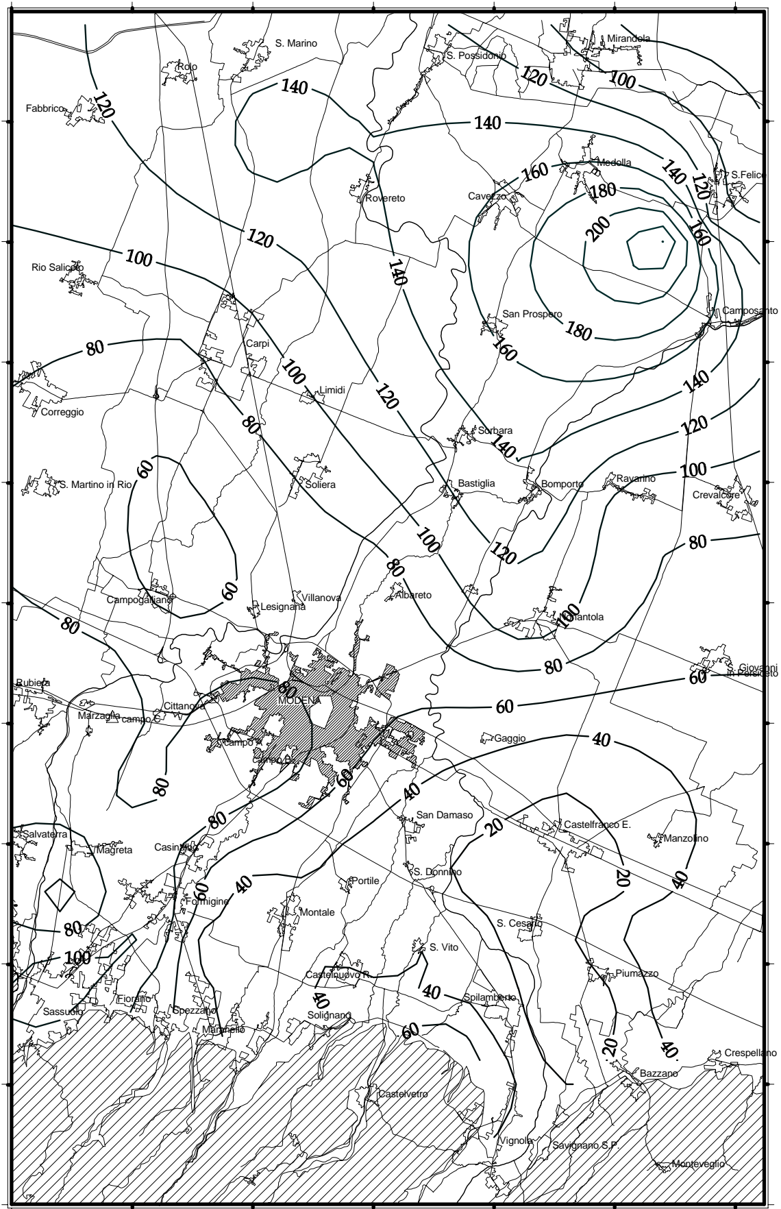
Figura 21 - Sodico (mg/l) media anno 2004.
