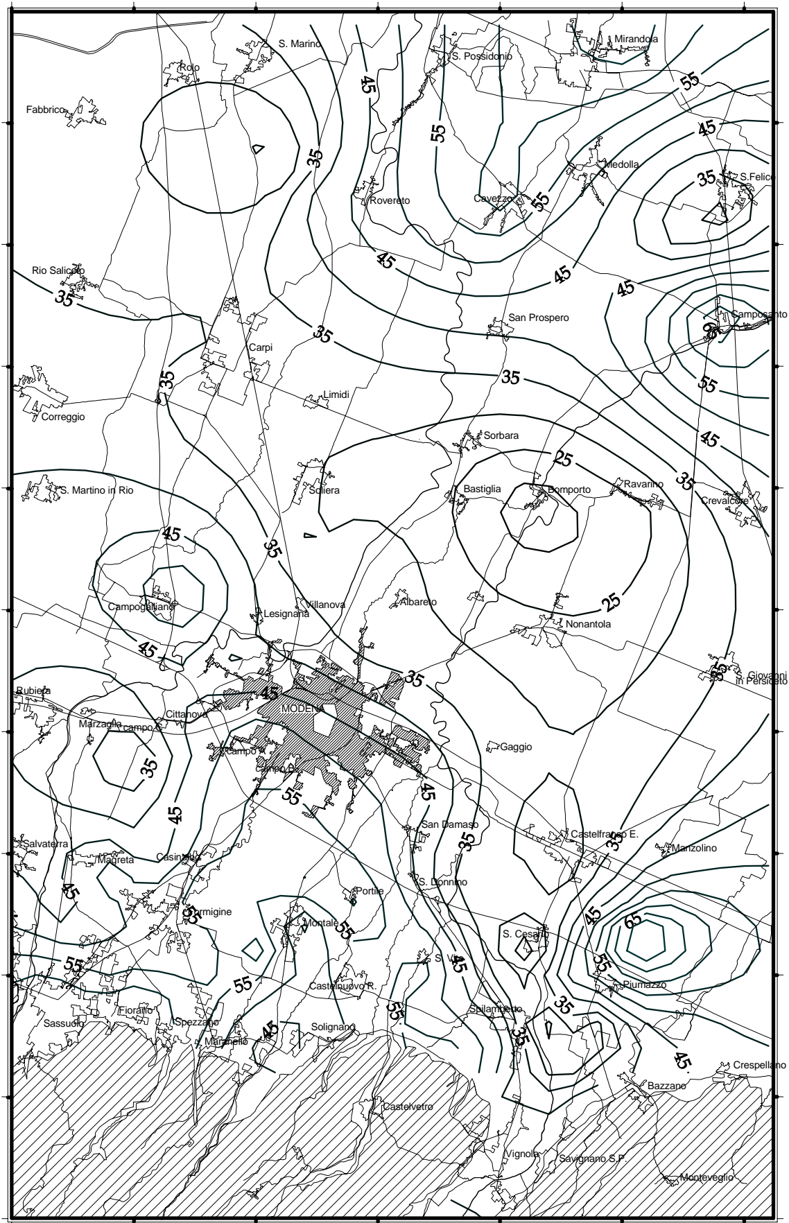
Figura 18 - Durezza (°F) media anno 2004.
