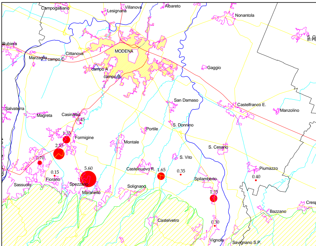
Figura 33 - Tricloroetilene media anno 2004.
