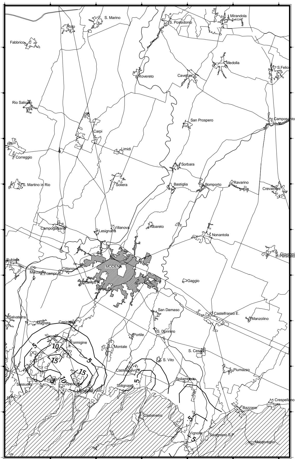
Figura 32 - Composti organo-alogenati totali ( \mu\text{g}/\text{l} ) media anno 2004.
