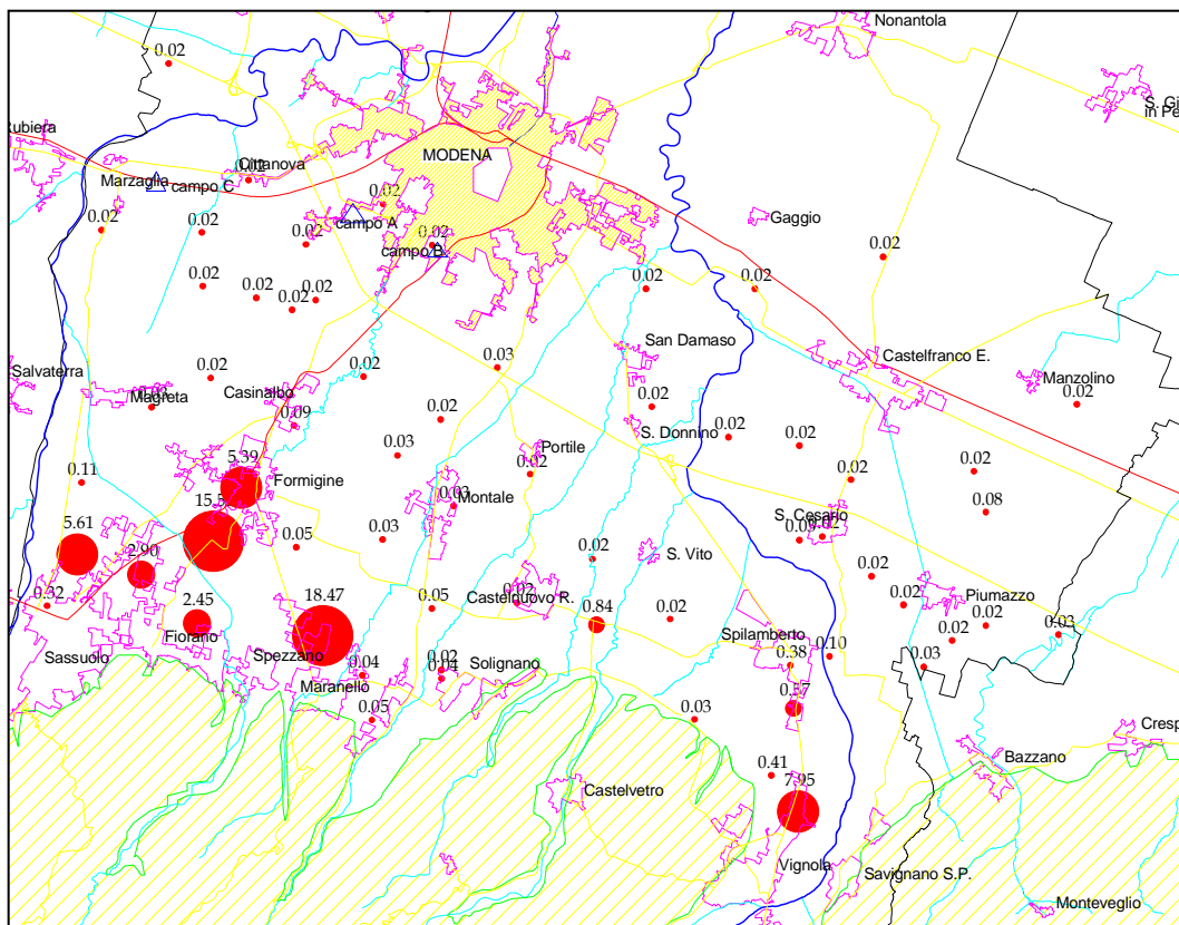
Figura 34 - Tetracloroetilene media anno 2004.
