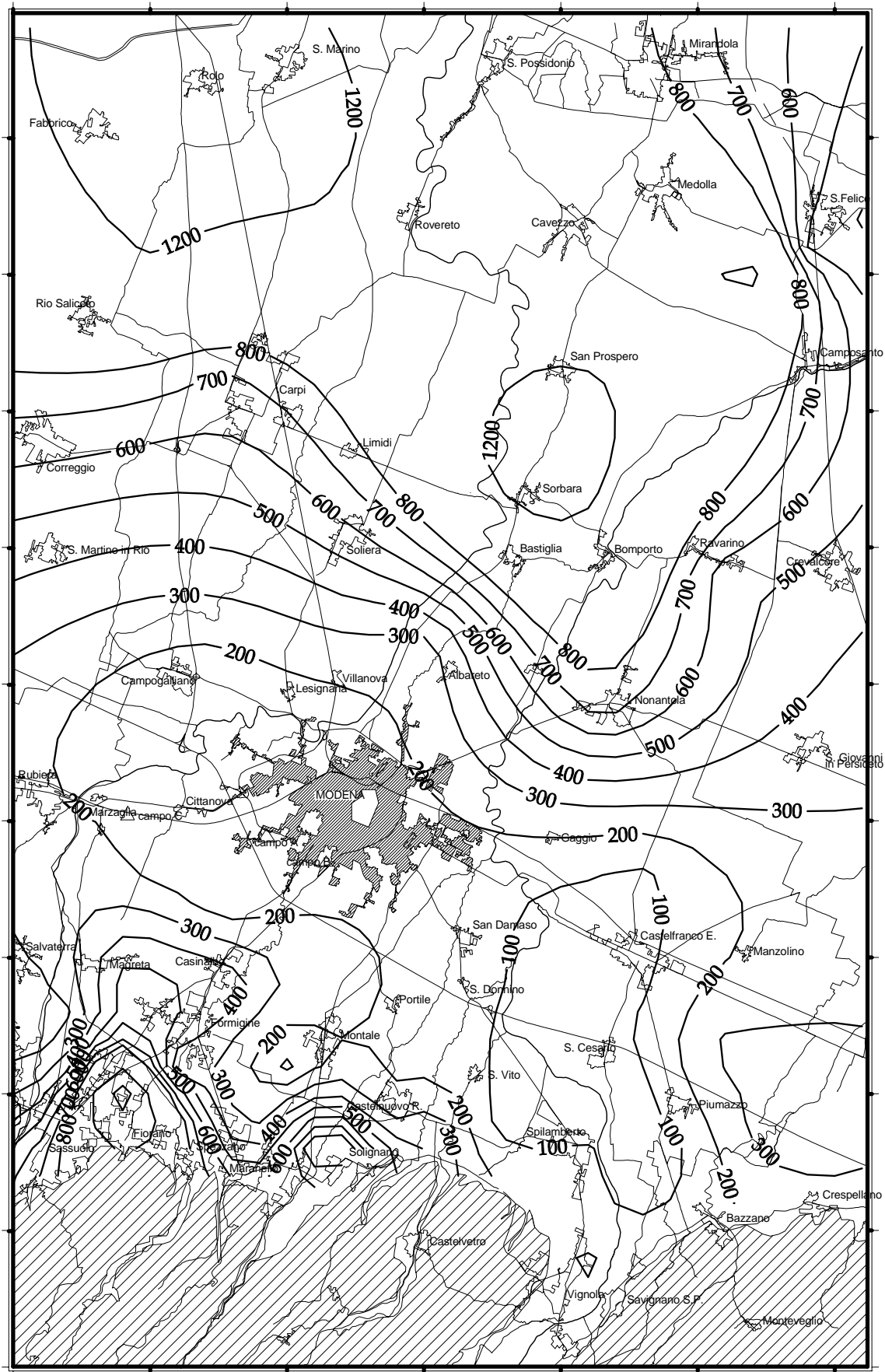
Figura 31 - Boro ( \mu\text{g/l} ) media anno 2004.
