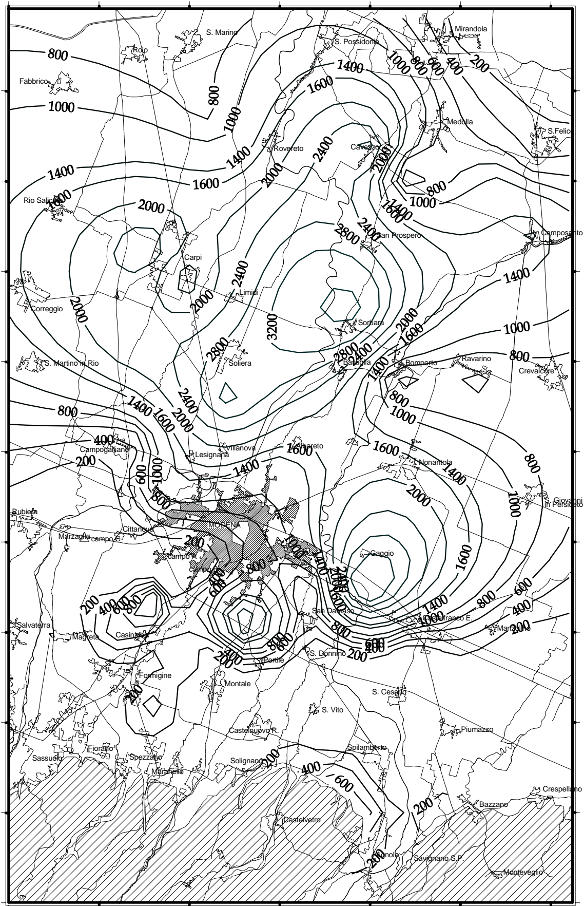
Figura 29 - Ferro ( \mu\text{g/l} ) media anno 2004.
