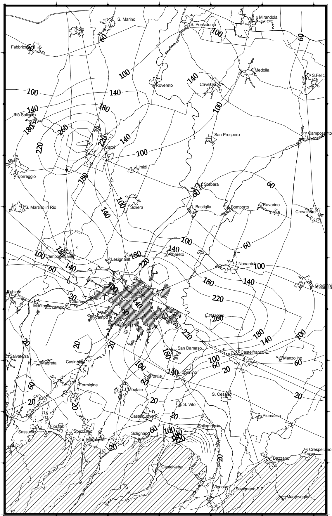
Figura 30 - Manganese ( \mu\text{g/l} ) media anno 2004.
