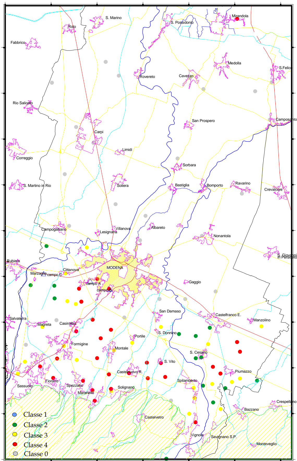
Figura 35 - Classificazione chimica anno 2004.
